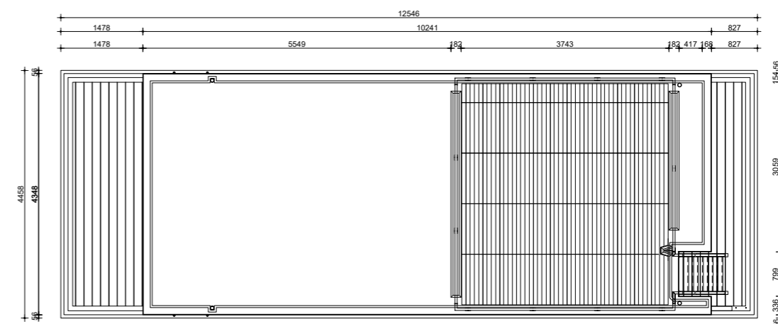
GRUNDRISS OBERDECK
