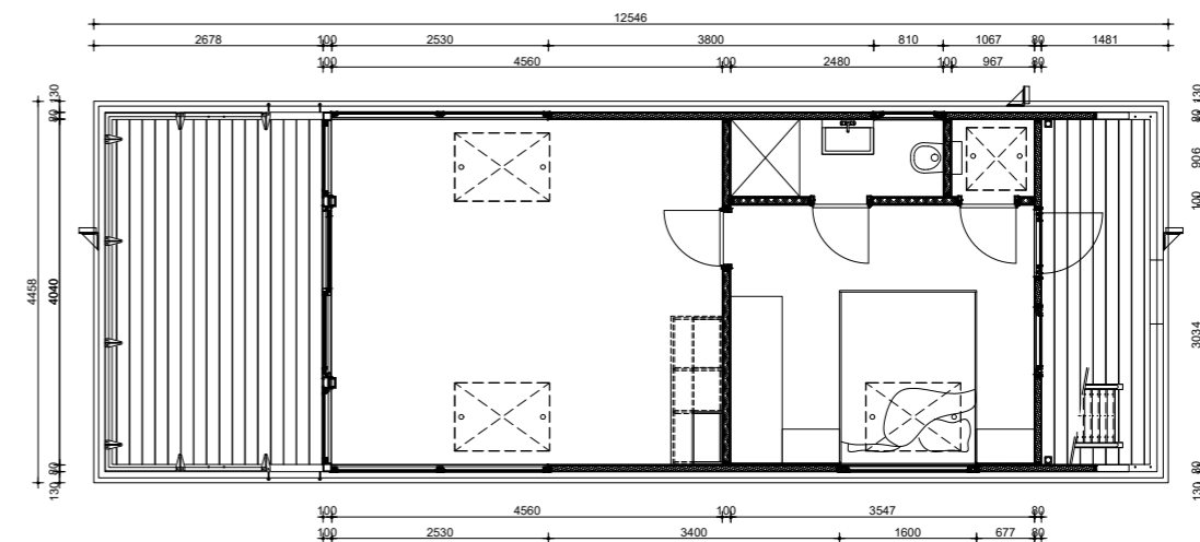
GRUNDRISS HAUS
